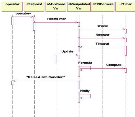
그림 12 시간 구동 조작 변수의 인터랙션 다이어그램
