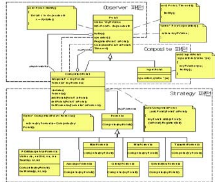
그림 3 포인트 클래스의 설계
