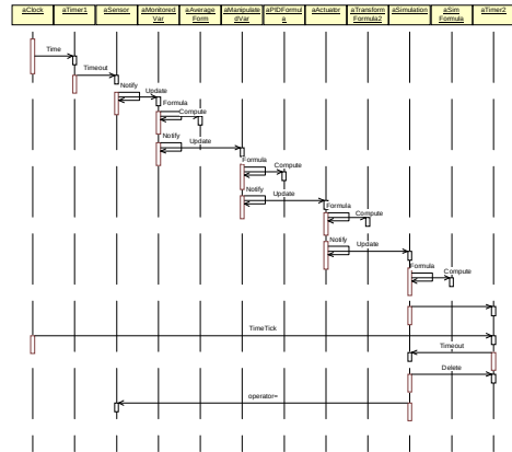
그림 19 방안 온도제어 루프 시스템의 인터랙션 다이어그램
