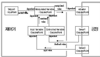
그림 9 전형적인 제어 루프 시스템의 구조
