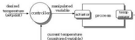
그림 17 방안 온도 제어 루프
