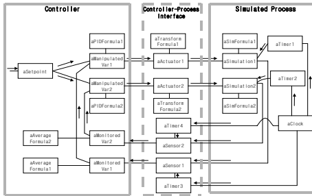
그림 22 복수의 공정 변수들을 갖는 제어 루프 어플리케이션의 객체 구조
