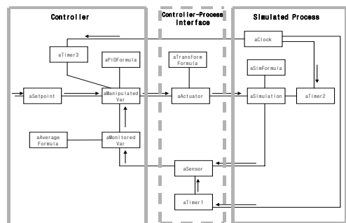
그림 18 방안 온도 제어 샘플 어플리케이션의 구조
