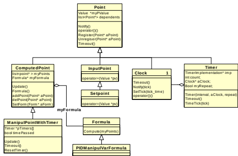
그림 11 클락 및 타이머 클래스와 조작 변수 클래스의 설계
