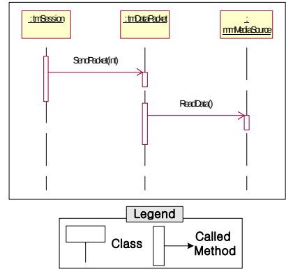
그림 7 데이터 패킷 송신시의 UML 시퀀스 다이어그램
