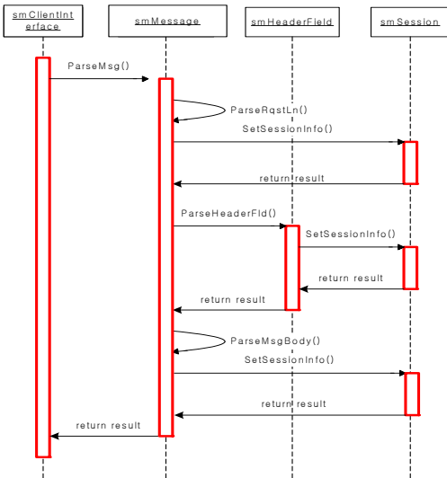
그림 21 메시지 해석 시퀀스 다이어그램
