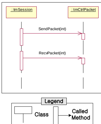
그림 9 제어 패킷 송신시의 UML 시퀀스 다이어그램
