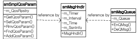
그림 23 승인 제어 클래스 모듈의 클래스 다이어그램
