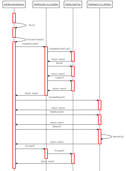
그림 17 서버 인터페이스에서 사용자 요구의 응답 처리 준비를 위한 시퀀스 다이어그램
