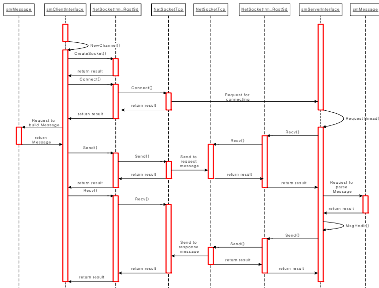
그림 18 클라이언트와 서버간의 메시지 전송 및 처리 시퀀스 다이어그램
