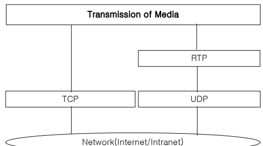
그림 4 전송관리자의 전송프로토콜 스택
