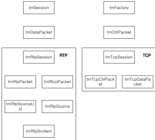
그림 11 전송관리자의 전체 모듈 구성도
